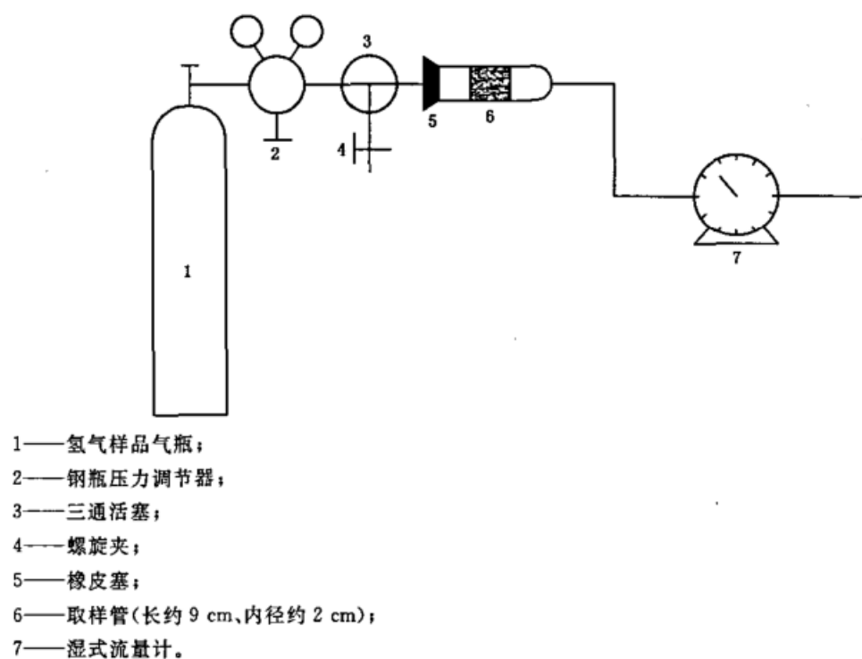
图 B.1 氯、碱测定装置示意图
